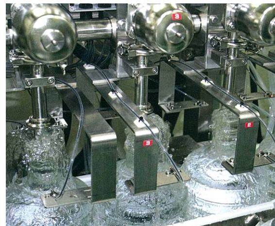
<充填機>
